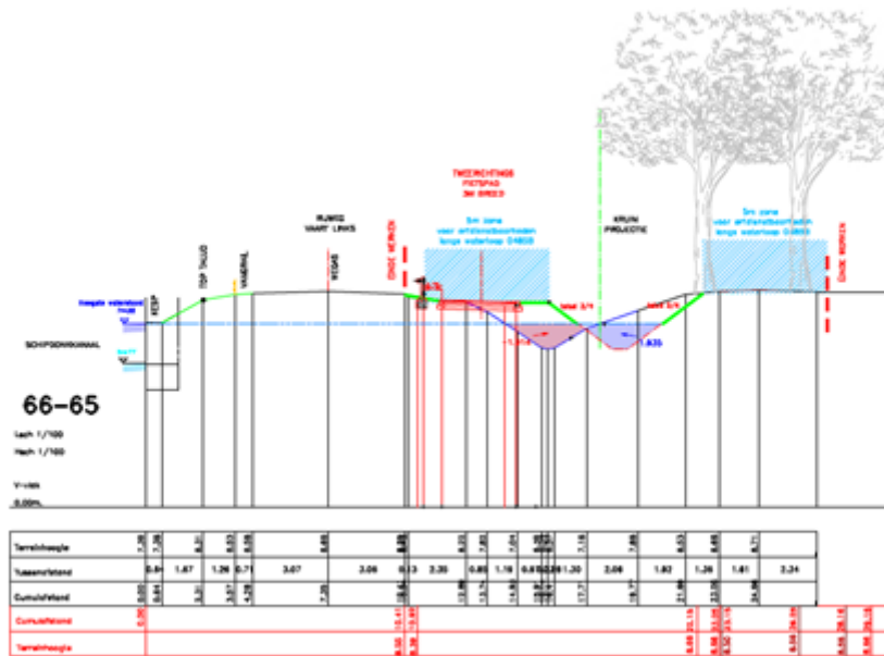
Dwarsprofiel scenario fietspad aanliggend aan de rijweg
