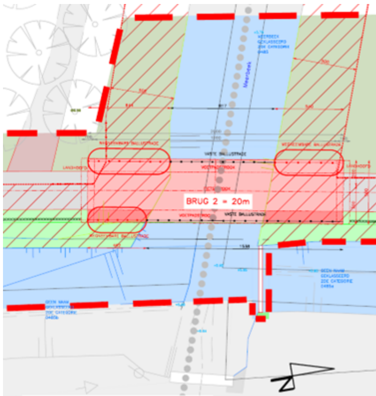
Detailtering wegneembare borstwering overbrugging 2 (zie onderstaande figuur):
